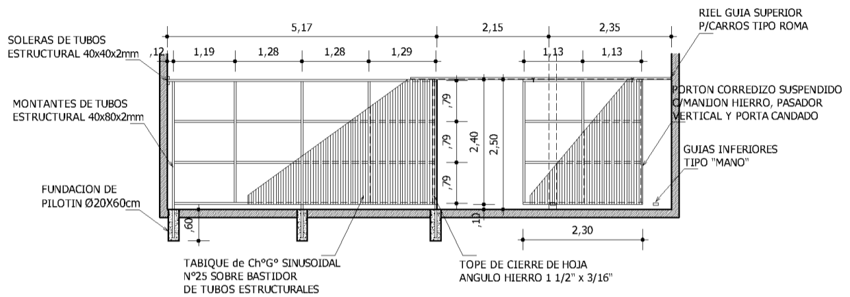
TABIQUE DE CERRAMIENTO VISTA FRONTAL - SIN ESCALA
