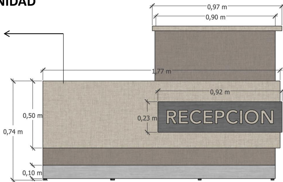
FRENTE
