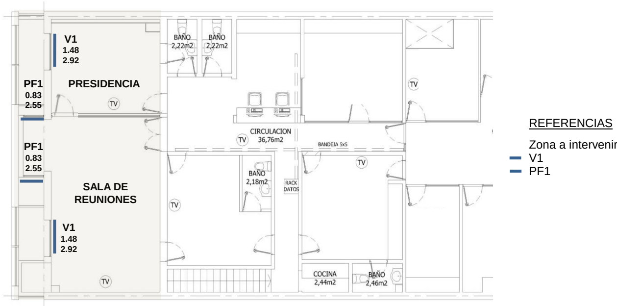
EDIFICIO CENTRAL GÜEMES N°45 - PRIMER PISO NOTA: todas las medidas deben ser verificadas en obra
