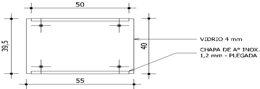
VISTA POSTERIOR PLEGADO CHAPA A° INOX. 1,2 mm
