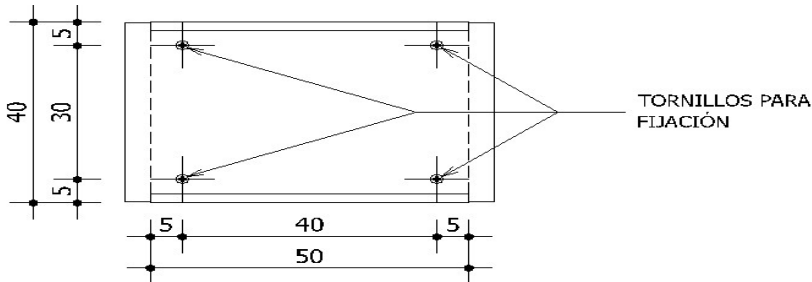
VISTA FRONTAL PLEGADO CHAPA A° INOX. 1,2 mm
